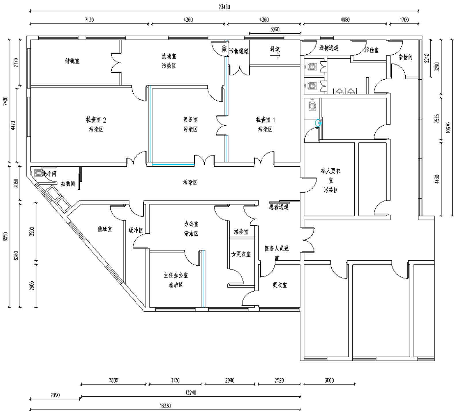
平面布置图 1:100
