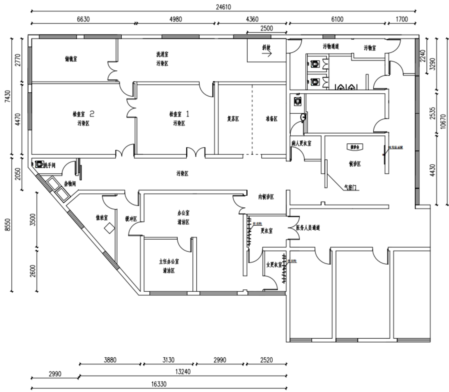
平面布置图 1:100
