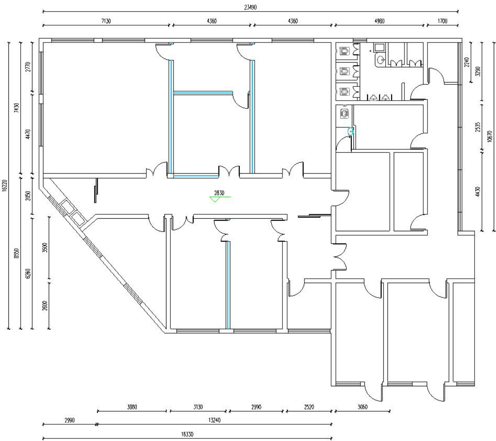
原平面图 1:100
